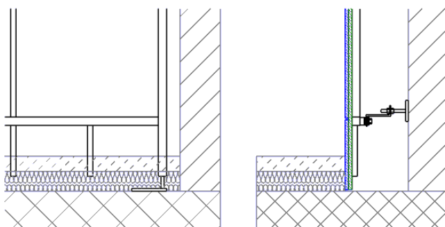
Bodenanschluss
